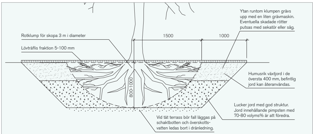
Figur 3. Detaljerad principskiss för trädgröp och växtbädd på den nya växtplatsen. Exempel för träd med stamomfång 70–120 cm. Illustration: Örjan Stål och SWECO.
